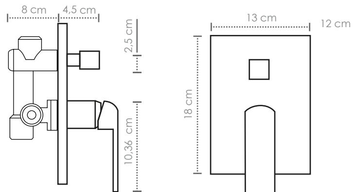
Alzado Lateral
